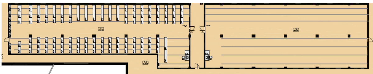
Dispozice - sklad C vlevo (zakresleno provizorní vybavení stacionárními regály), sklad E vpravo
